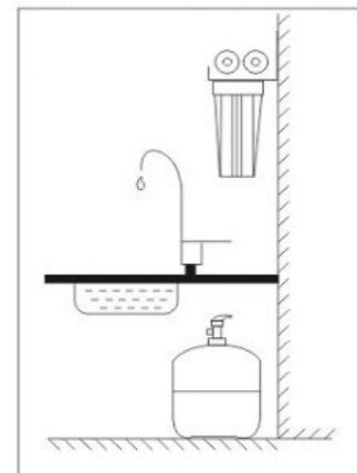
Fig. 8: Montaje de pared
