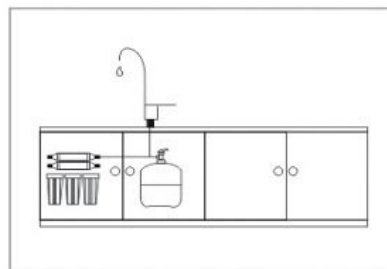
Fig. 7: Debajo de la encimera
