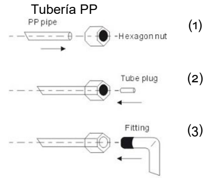
Fig. 16: Conector rápido manguera PE
