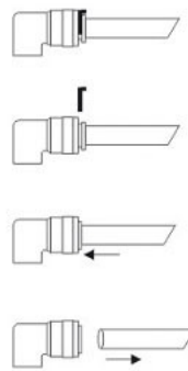
Fig. 15: Separación conector rápido manguera PE
