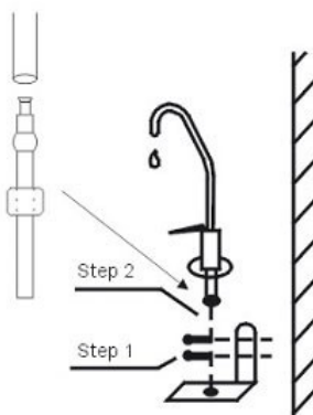
Fig. 9: Grifo de pared
