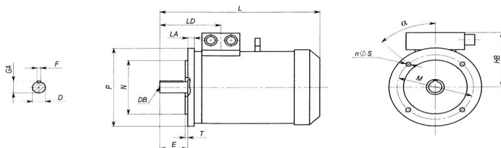
Bride B5
