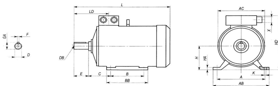
Bride B3
