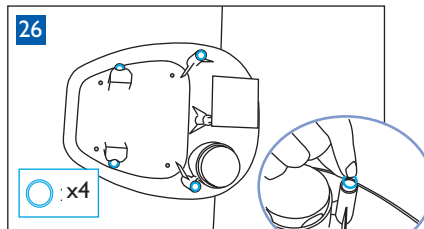
Mettez obligatoirement en place les 4 petits joints (inclus dans le kit de fixation).
