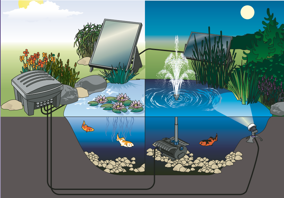
Représentation schématique : Aquarius Solar en combinaison avec d'autres composants solaires OASE
