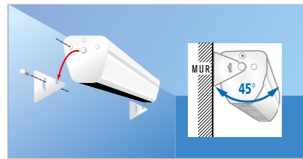
>Pose et réglage au mur
