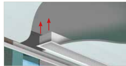
>Pose et réglage au plafond sur le bati
