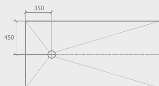
Position de l'écoulement sur receveur 1800 x 900 mm
