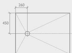
Position de l'écoulement sur receveur 1200 x 900 mm
