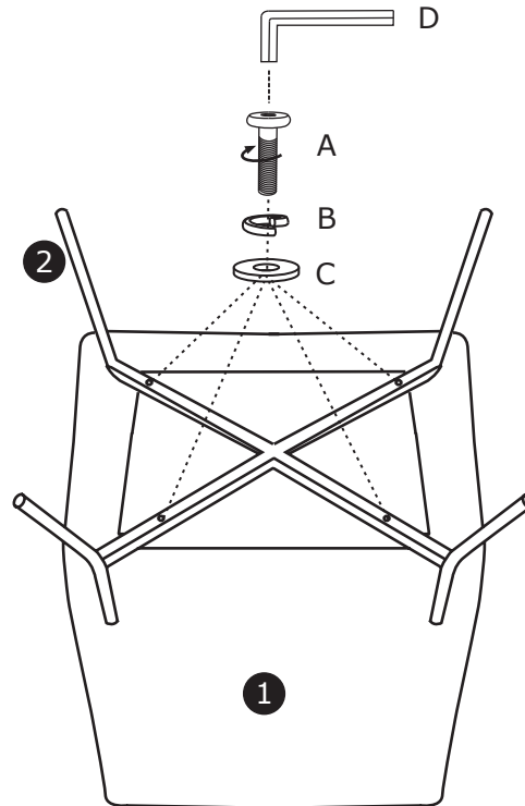
M6x11mm Bx4
