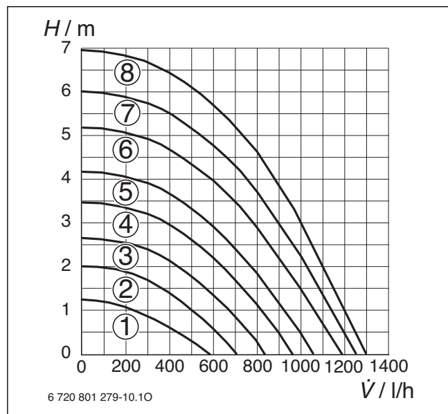
Fig. 65 Courbes caractéristiques de pompe pour les appareils ZSBR
