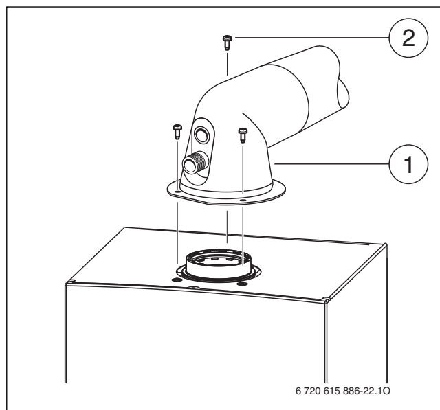
Fig. 35 Fixer la ventouse
