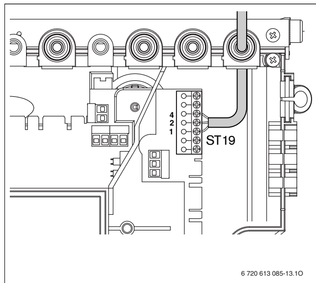
Fig. 41 Raccordement 24 V
