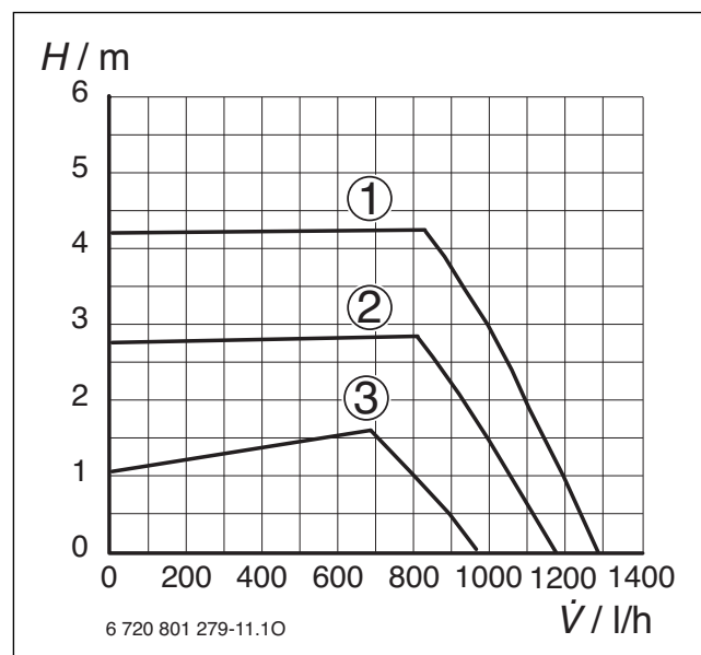
Fig. 63 Pression constante
