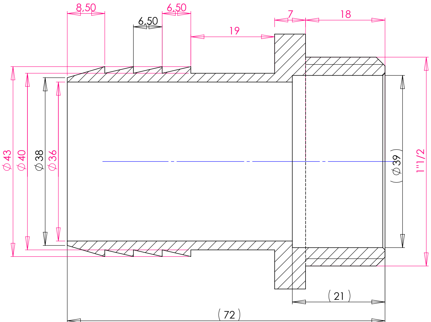
B-B (2 : 1)
