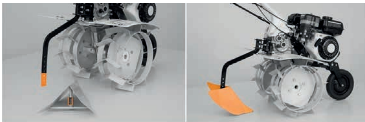
Positionner le buteur et serrer avec une vis
