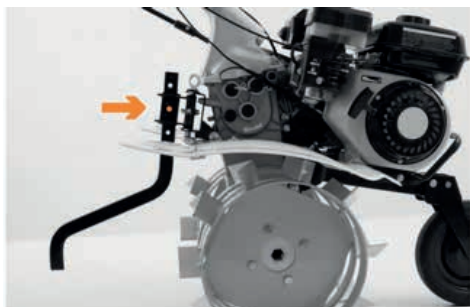
Enlever le pic terrage
