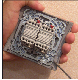
1. Démontez la plaque à l'aide d'un tournevis aux 4 coins du produit
