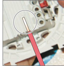
2. Mesurer la longueur des fils à dénuder en utilisant le gabarit intégré au produit
