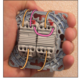
3. Enfiler les fils dans les bornes auto-serrantes (Pour ôter les fils, exercer une pression avec le doigt sur les languettes).
