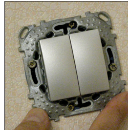
4. Dévisser légèrement les 2 vis de la boîte d'encastement pour permettre le passage des 2 têtes de vis
