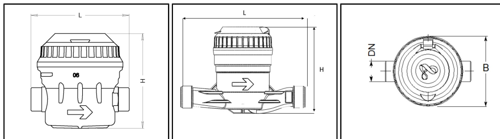
DN 15 - vue de face
