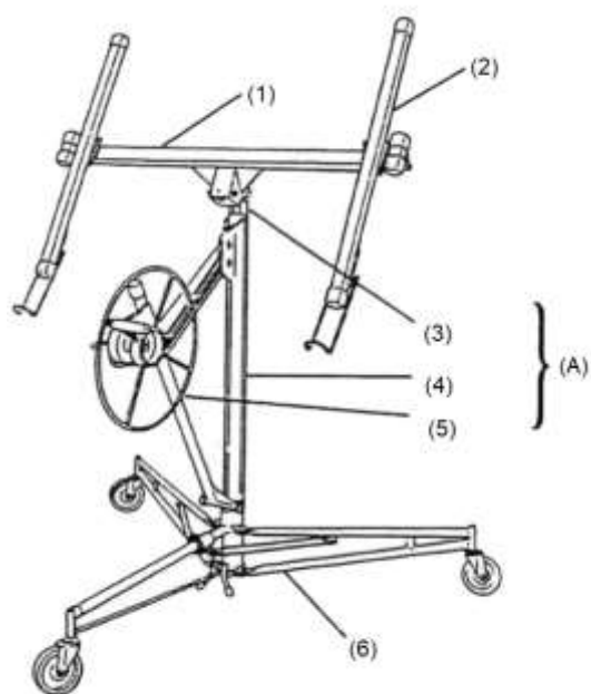
Composants du lève-panneaux
