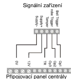
Připojovací panel centrály
