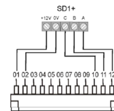
Připojovací panel centrály
