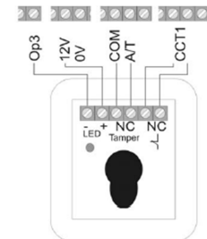
Připojovací panel centrály
