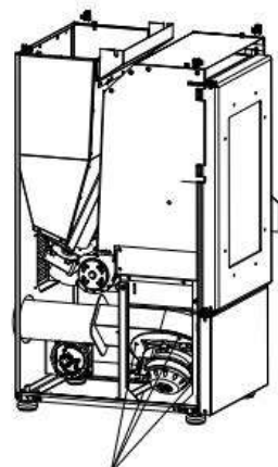
Scollegare il filo dal ventilatore di scarico fumi e utilizzare una chiave a brugola da 4 mm per svitare la vite di fissaggio e rimuoverla per la pulizia
