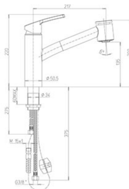
Schéma technique
