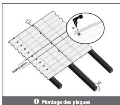
1 Montage des plaques
