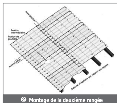
2 Montage de la deuxième rangée
