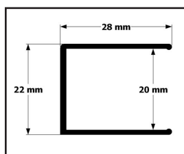
Profilo muro lato porta
