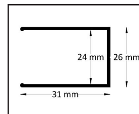
Profilo muro vetro fisso
