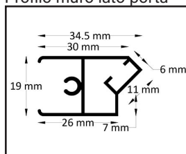
Profilo riscontro calamita
