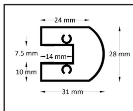
Profilo vetro rotante
