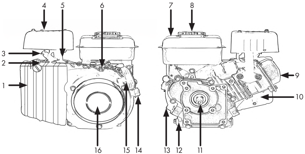
Figuur 1: Algemene onderdelen van de benzinemotor
