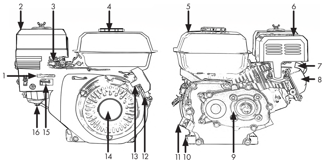
Figur 1: Bensinmotorns allmänna komponenter
