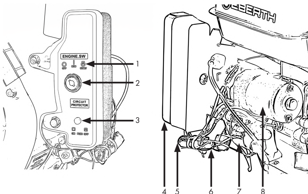
Figura 3: Dettagli sui motori con E-Start
