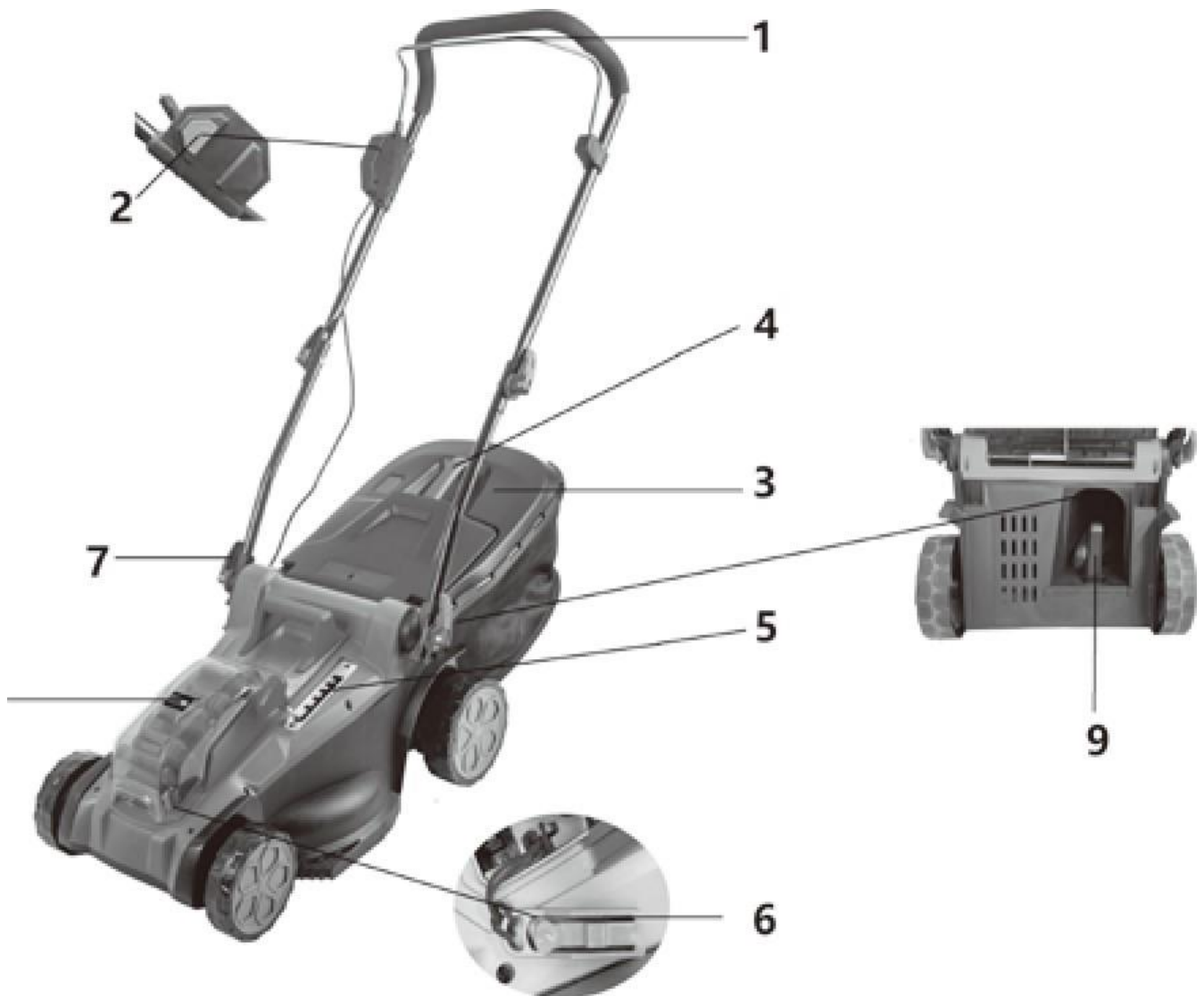
Abbildung 1: Rasenmäher
