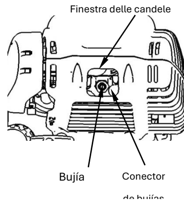
Extracción de bujías
