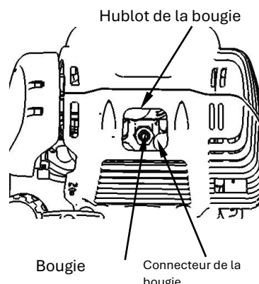
Démontage bougie
