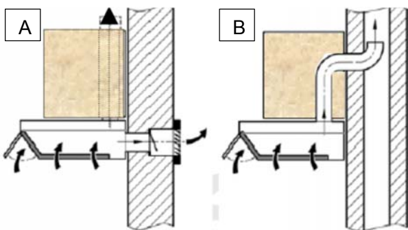
Fig. B Abluft über einen Luftschacht
