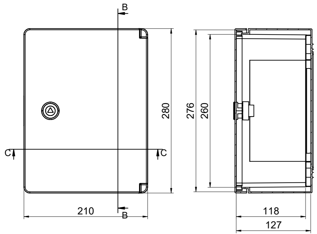
B-B
