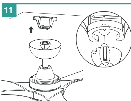
11 Hang the ceiling fan. Cuelgue el ventilador. Accrochez le ventilateur de plafond.
