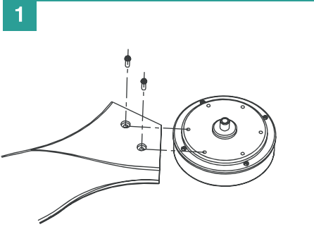
1 Blade assembly. Monte las palas. Assemblage de les lames.
