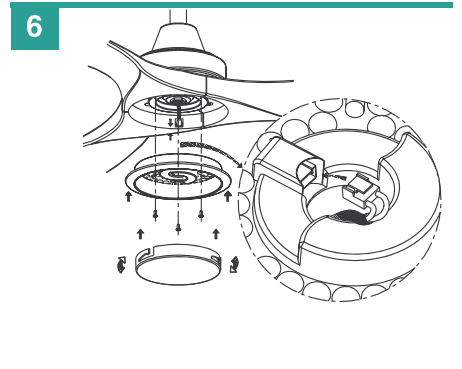
6 Connect the light kit and twist the diffuser. Conecte el kit de luz y enrosque el difusor. Connectez le kit d'éclairage et tournez le diffuseur.
