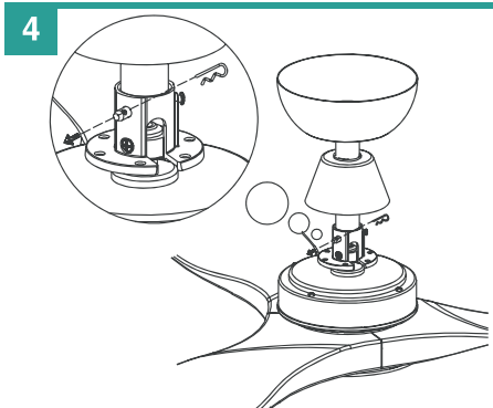
4 Secure the pin by insert the stop pin. Coloque el gancho en el extremo del pasador. Lors de l'insertion du croisillon
