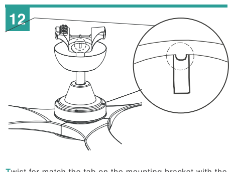
12 Twist for match the tab on the mounting bracket with the ball slot on the ball. Gire el conjunto de ventilador para hacer coincidir la lengüeta del soporte con la ranura de la bola. Tournez pour faire correspondre la languette du support de montage avec la fente de balle sur la balle.
