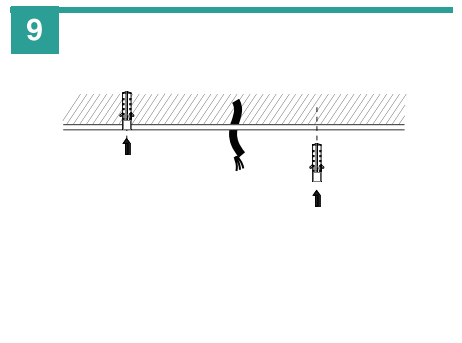
9 Place de wall plugs. Inserte los tacos. Installez les chevilles.
