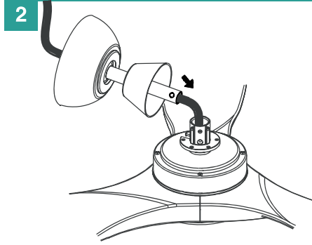
2 Thread the power leads from the fan through the down rod. Pase los cables por la tija. Passez les fils à travers la tige.
