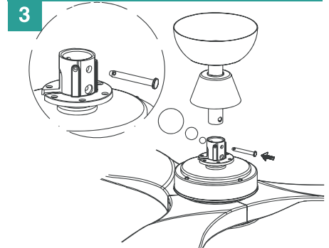
3 Put the downrod to the motor and the connecting pin. Pase los cables a través de la tija y coloque el pasador. Insérer les fils du moteur au travers la tige. Insérer la croisillon
