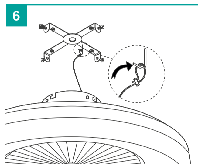
6 Hang the fan on the hook. Cuelgue el ventilador. Accrochez le ventilateur de plafond au crochet.
