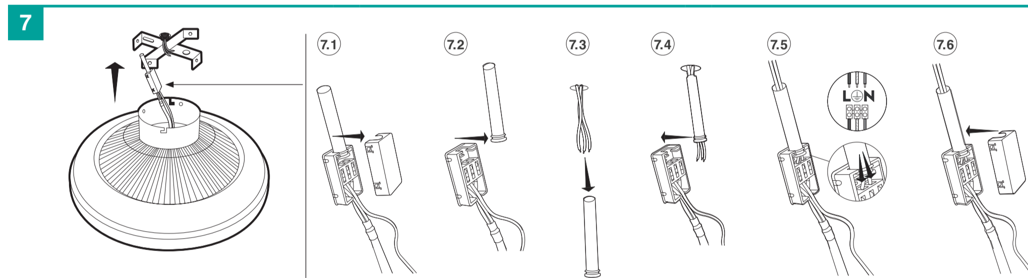
7 Make the connections. Haga las conexiones. Si tiene dudas consulte a un técnico. Faites les connexions. En cas de doute, consultez un technicien.
