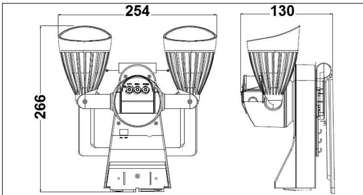
Fig.4 – DIMENSIONS / DIMENSIONI (AVEC détecteur / CON rilevatore / WITH sensor)
