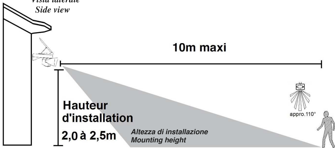
Fig.4 – DIMENSIONS / DIMENSIONI (AVEC détecteur / CON rilevatore / WITH sensor)
