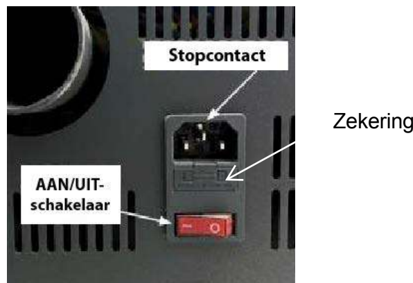
Aansluiting Voeding + AAN/UIT-schakelaar
