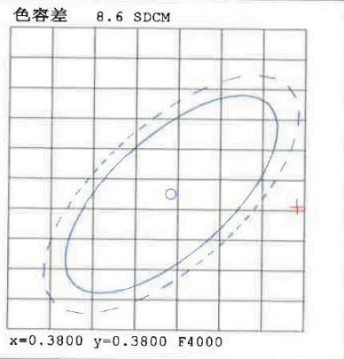
CIE1931色品图
