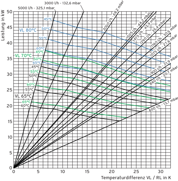
Leistungsdiagramm VIH R 300
