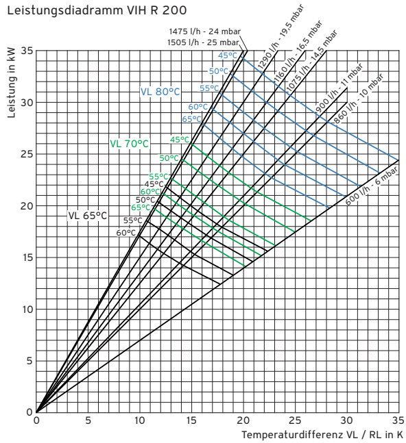
Leistungsdiagramm VIH R 200
