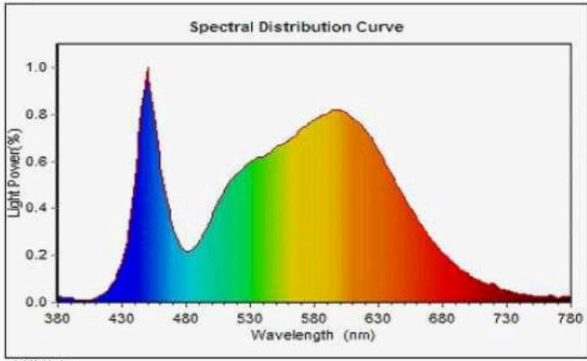
光谱分布
