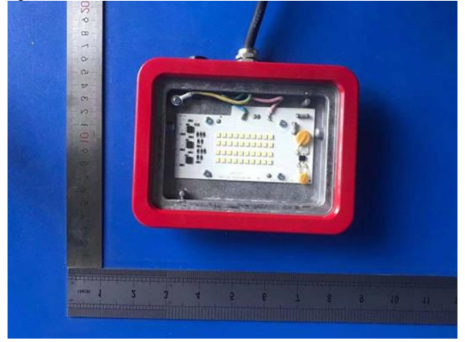
KCL01-30H
