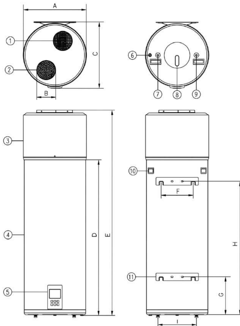
Abb. 3 Abmessungen des Geräts
