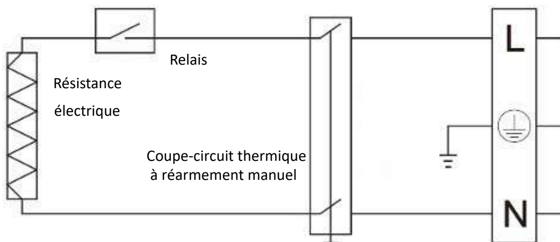
Fig. 2 Principe de fonctionnement du chauffage électrique d'appoint
