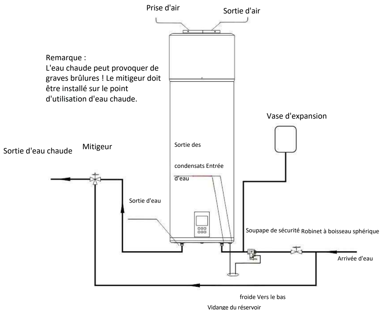
Fig. 6 Raccordement de la tuyauterie
