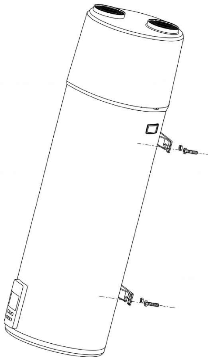
Fig. 4 Espace recommandé pour l'installation et la maintenance de l'appareil.
