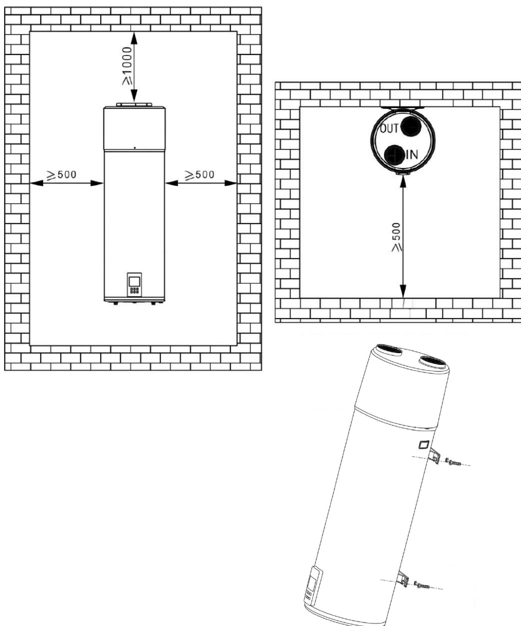
Fig.4 Espacio de instalación y mantenimiento recomendado
