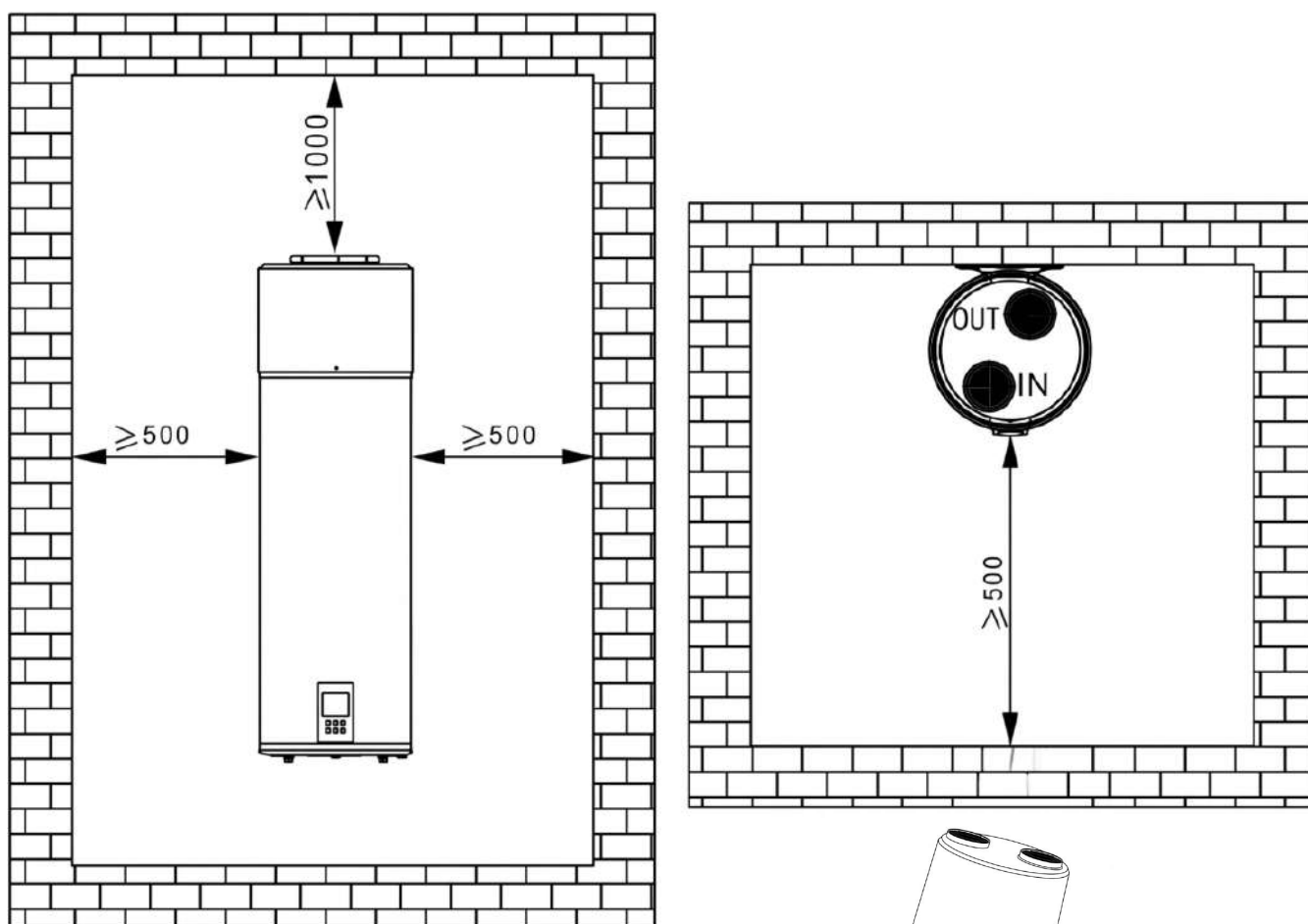
Rys. 4. Zalecana przestrzeń do instalacji i serwisowania
