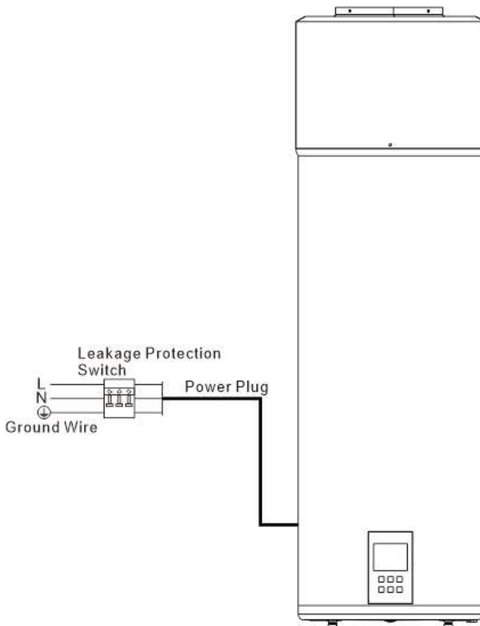
Fig. 8 Aardlekschakelaar
