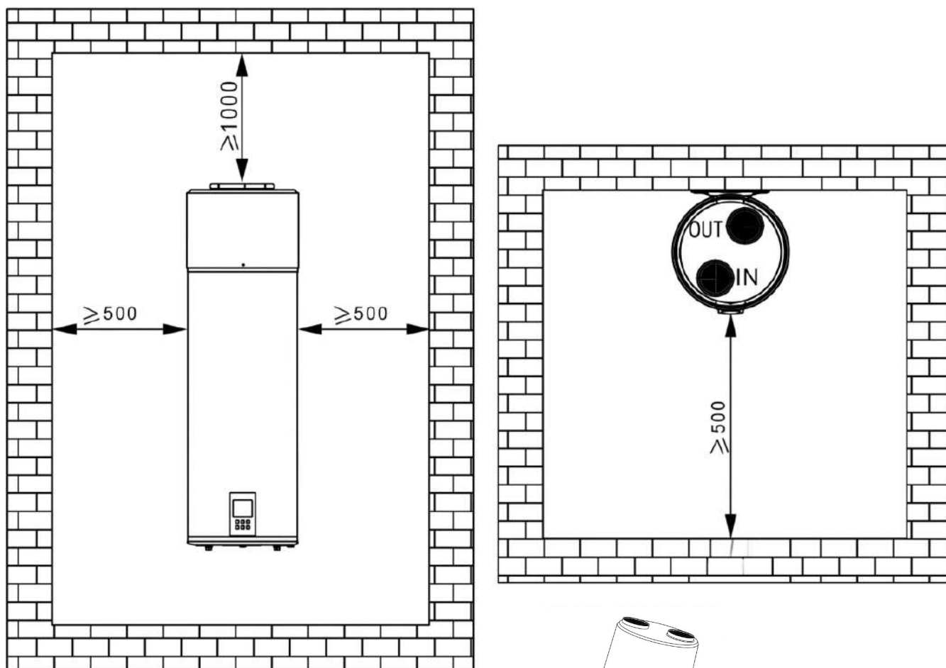
Fig.4 Distanze consigliate per l'installazione e la manutenzione dell'apparecchio
