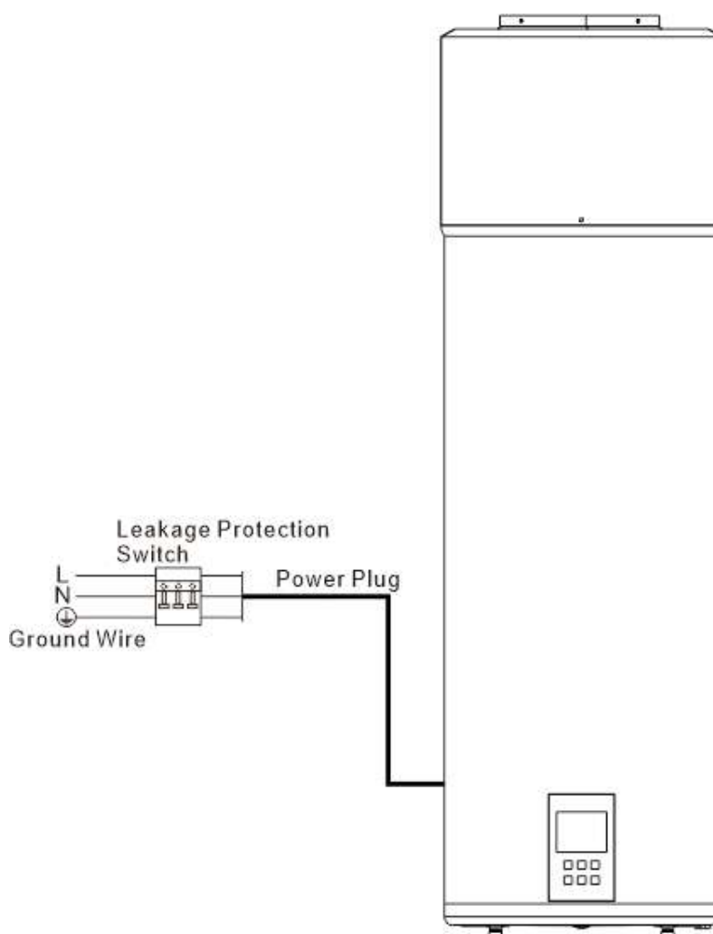
Fig.8 Protezione differenziale
