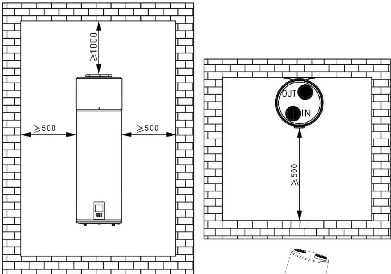
Fig. 4 Aanbevolen installatie- en onderhoudsruimte
