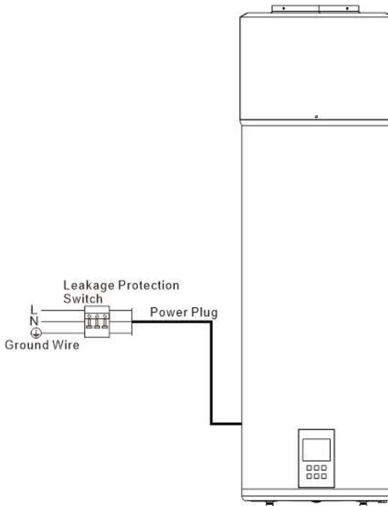
Obr. 8 Ochrana proti zemnímu spojení
