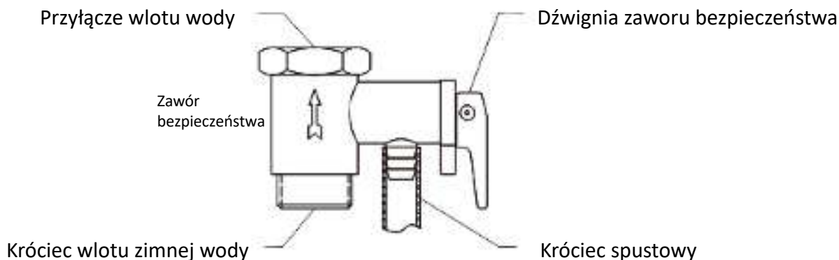
Rys. 8. Zawór bezpieczeństwa
