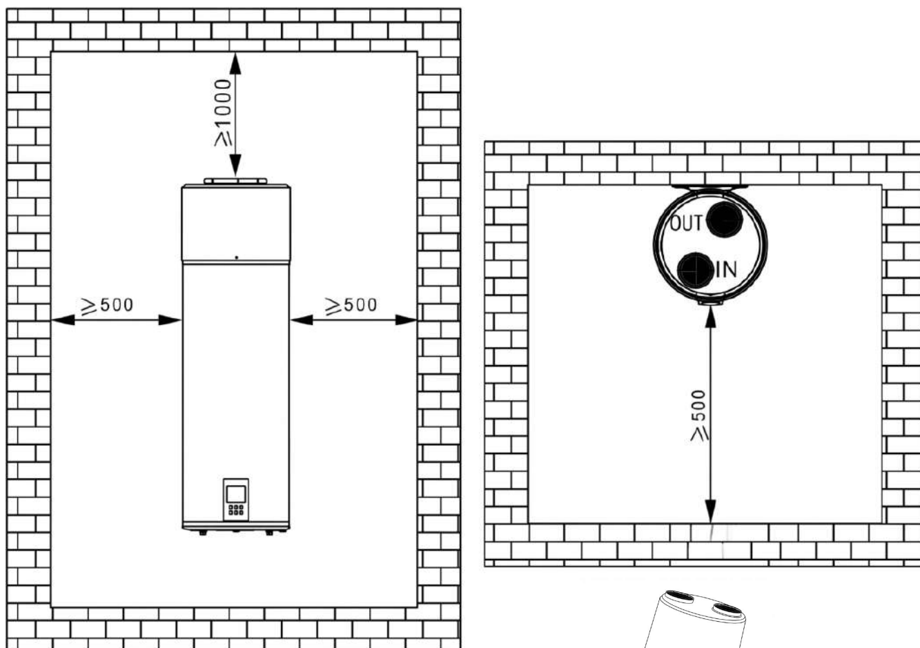
Fig. 4 Espaço recomendado para instalação e manutenção
