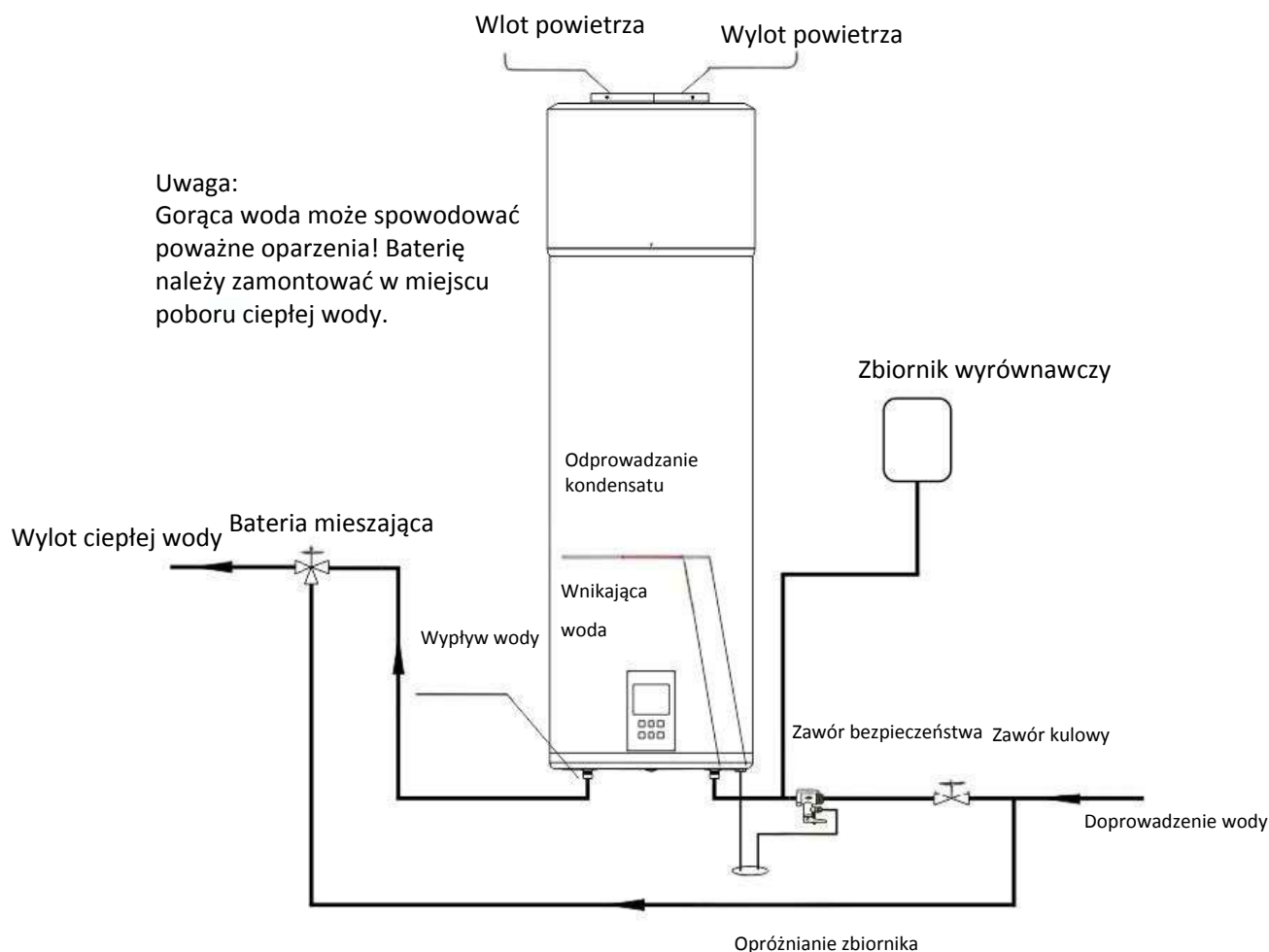
Rys. 6. Podłączenie instalacji rurowej
