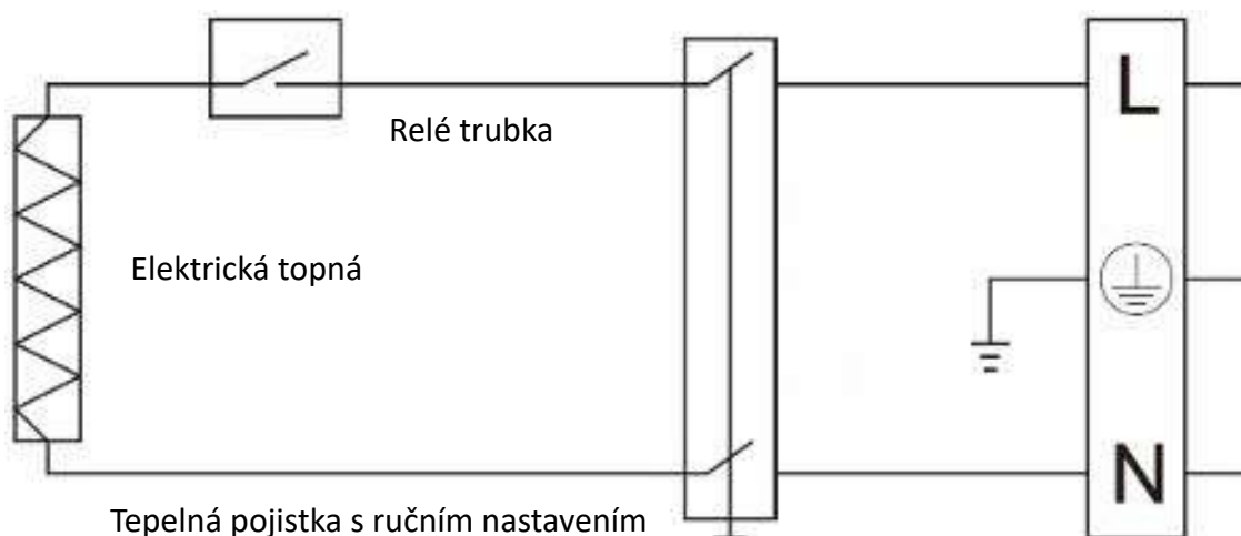
Obr. 2 Princip činnosti elektrického asistenta vytápění
