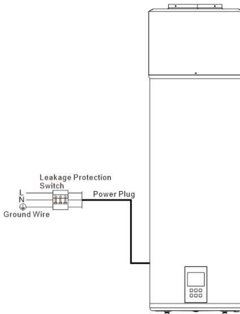
Fig. 8 Protection différentielle
