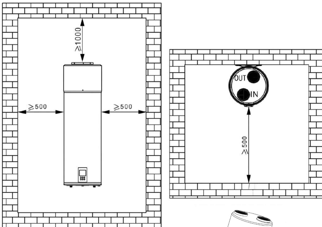
Obr. 4 Doporučený prostor pro instalaci a údržbu
