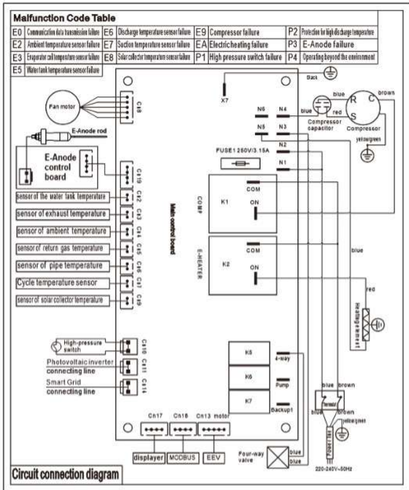
Fig. 9 Bedradingsschema
