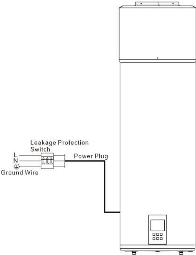
Fig. 8 Proteção de fuga à terra
