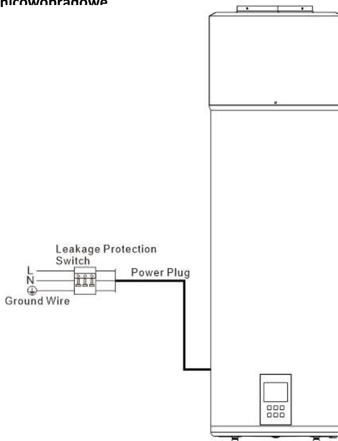
Rys. 8. Ochrona przed prądem upływowym
