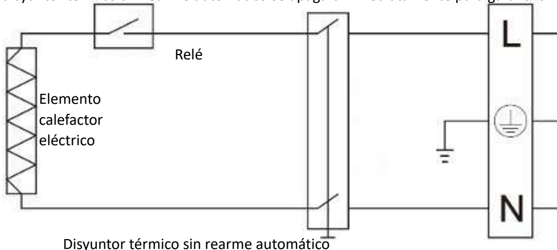
Fig. 2 Principio de funcionamiento del calentamiento asistido por electricidad
