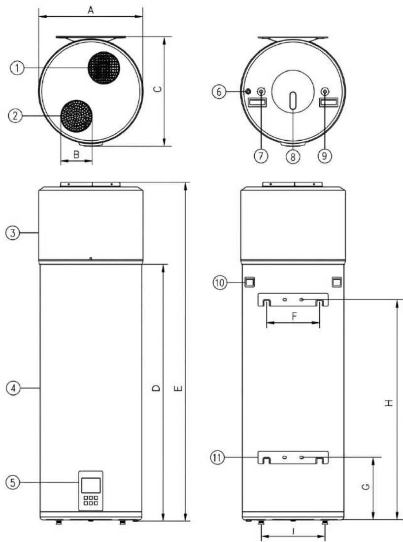
Fig. 3 Dimensiones del aparato
