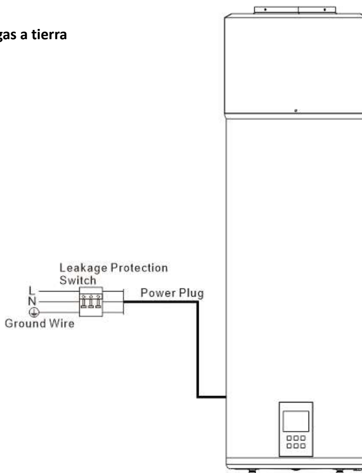
Fig.8 Protección contra fugas a tierra
