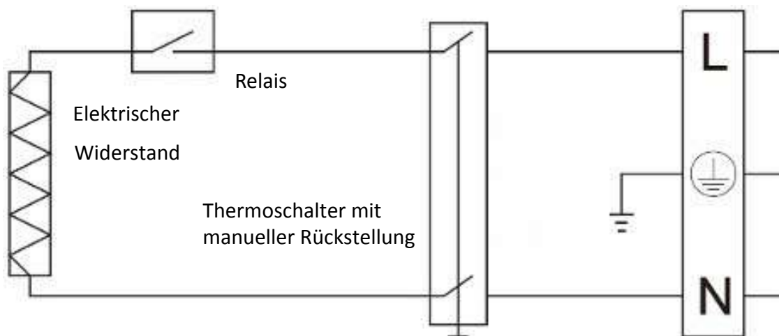
Abb. 2: Funktionsprinzip des elektrischen Zusatzheizstabs
