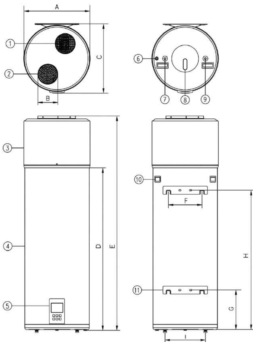
Fig. 3 Dimensões do aparelho
