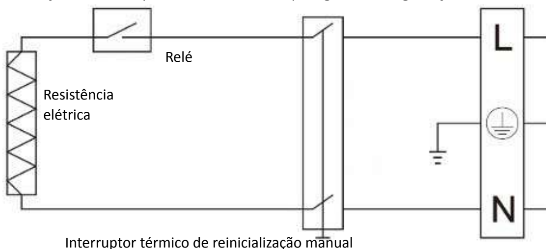
Fig. 2 Princípio de funcionamento do aquecimento assistido por eletricidade
