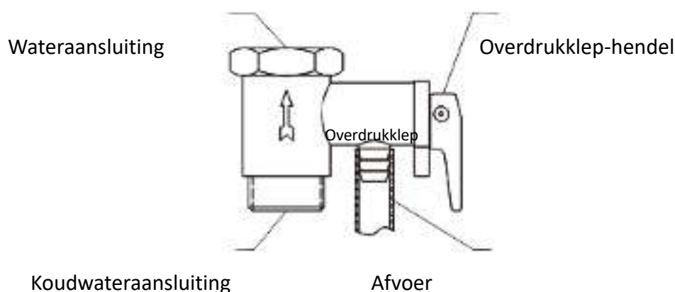
Fig. 8 Overdrukklep
