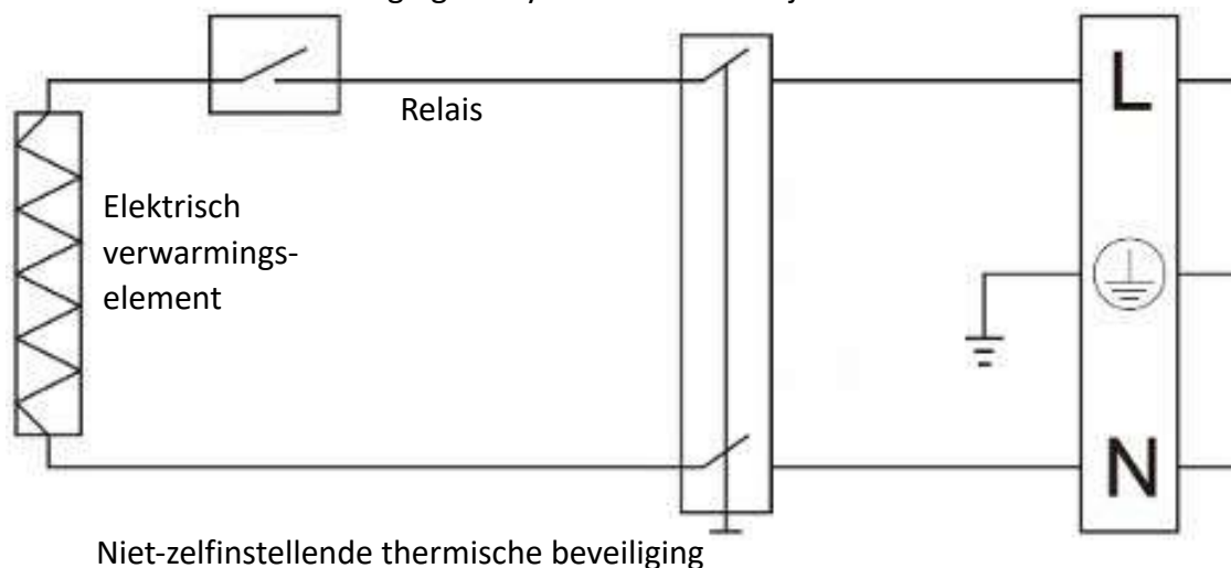
Fig. 2 Werkingsprincipe van elektrische bijverwarming
