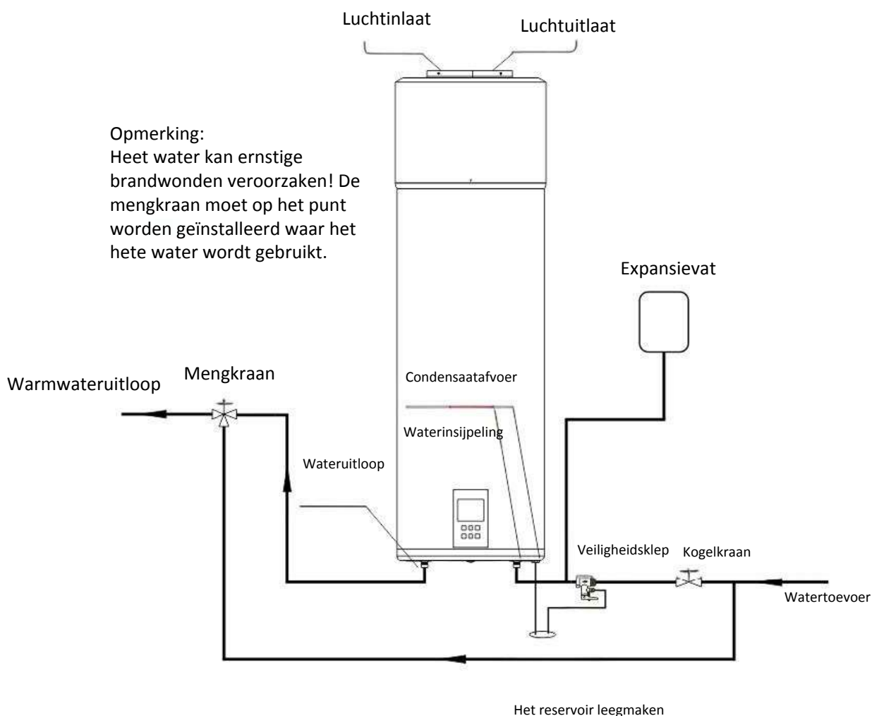
Fig. 6 Aansluiting leidingsysteem
