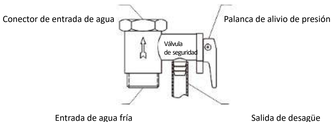
Fig.8 Válvula de seguridad
