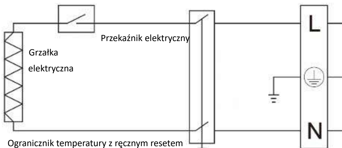
Rys. 2. Zasada działania funkcji dogrzewania elektrycznego
