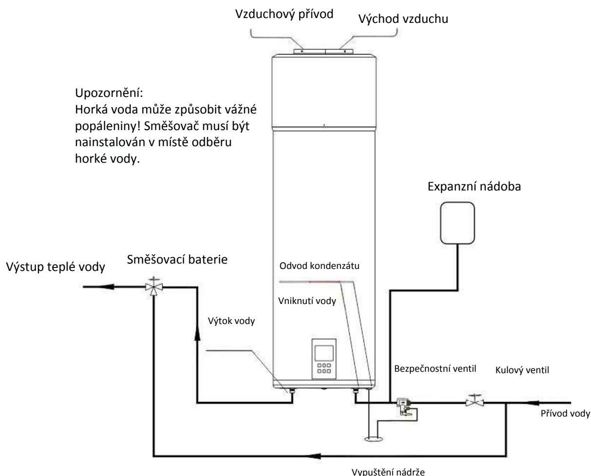
Obr. 6 Připojení systému potrubí
