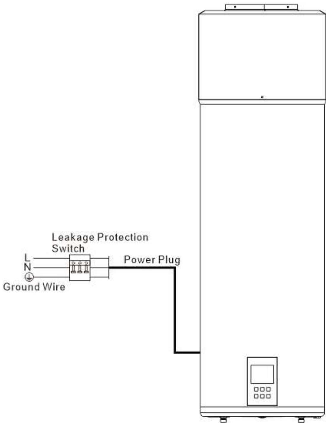
Abb. 8: Fehlerstromschutz
