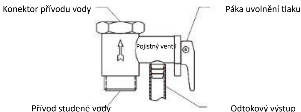
Obr. 8 Pojistný ventil
