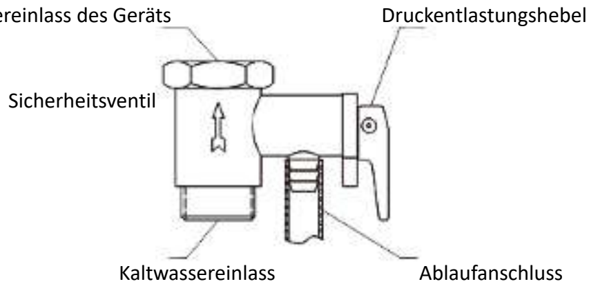
Abb. 8 : Sicherheitsventil
