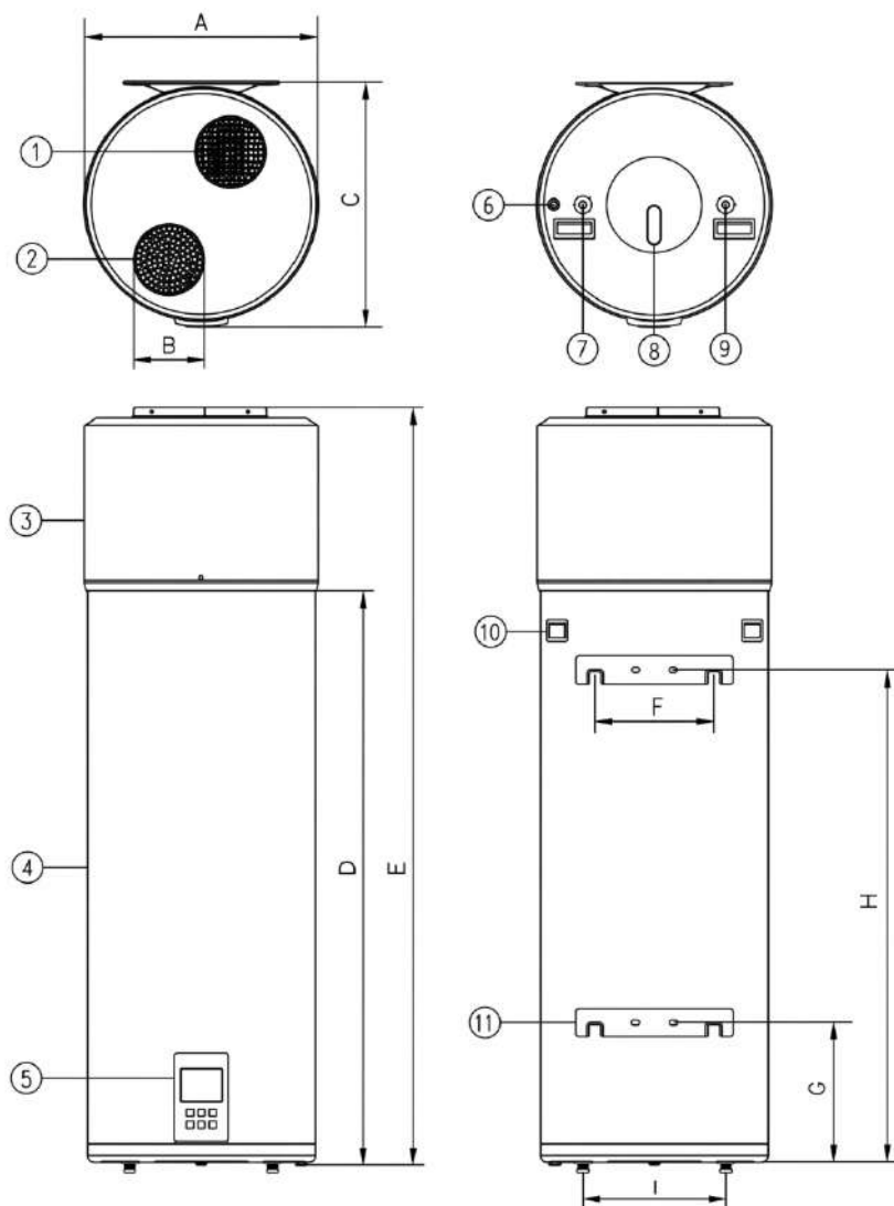
Afb. 3 Afmetingen van het apparaat
