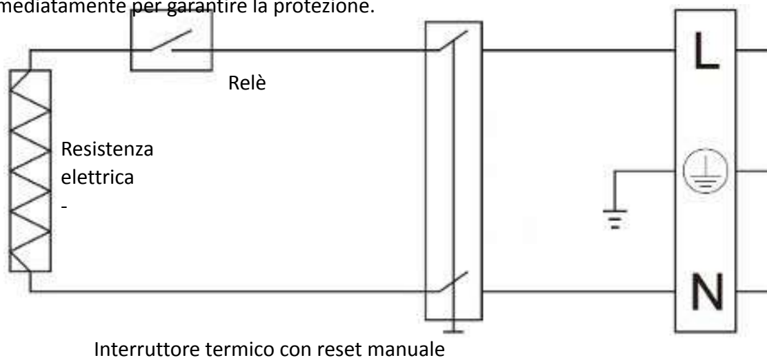
Fig. 2 Principio di funzionamento del riscaldamento elettrico ausiliario
