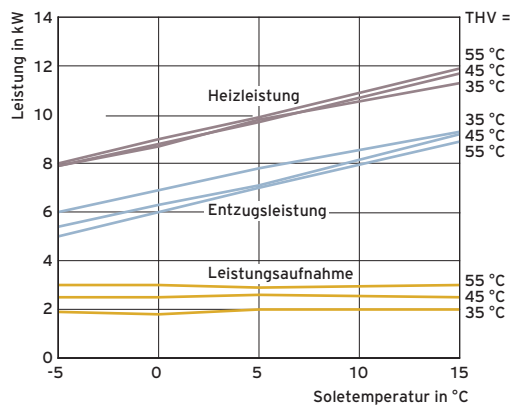
Leistungsdiagramm VWF 88/4
