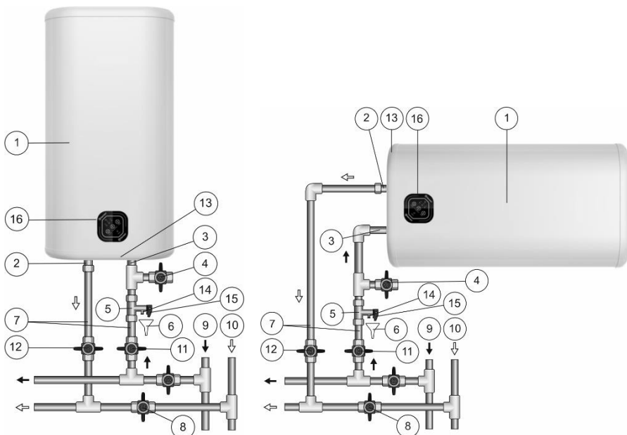
Figure 1. Schéma de connexion de CHE à la canalisation d'eau
